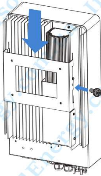
Встановлення підвісної панелі інвертора
